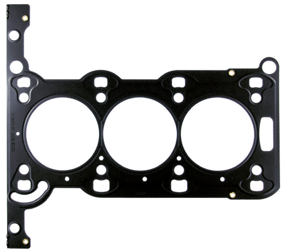
Ilustracja_Uszczelka głowicy cylindrów nr Reinz 61-33495
